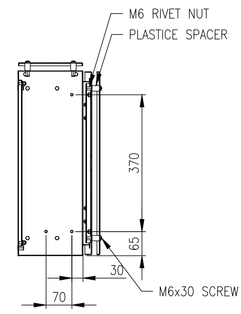
SECTION AV-AV
