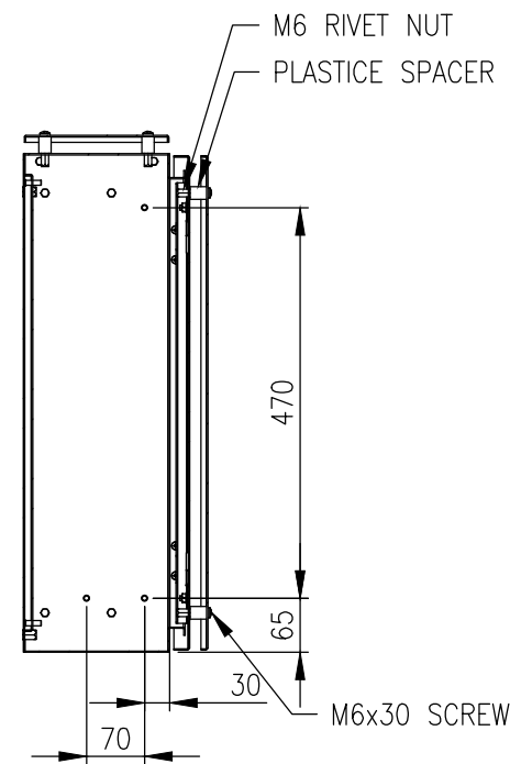
SECTION AV-AV
