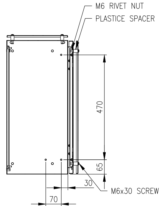
SECTION AV-AV
